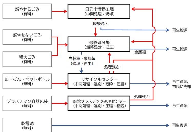
家庭系ごみの分別区分とごみ処理フロー
