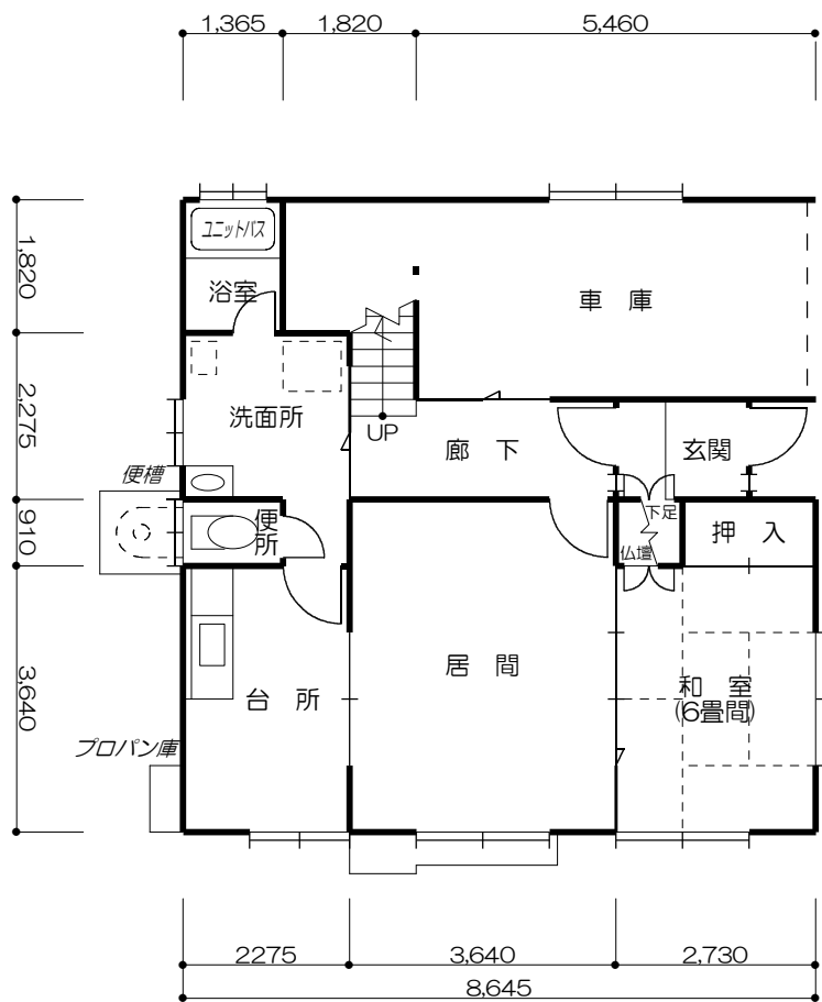
1階平面図
