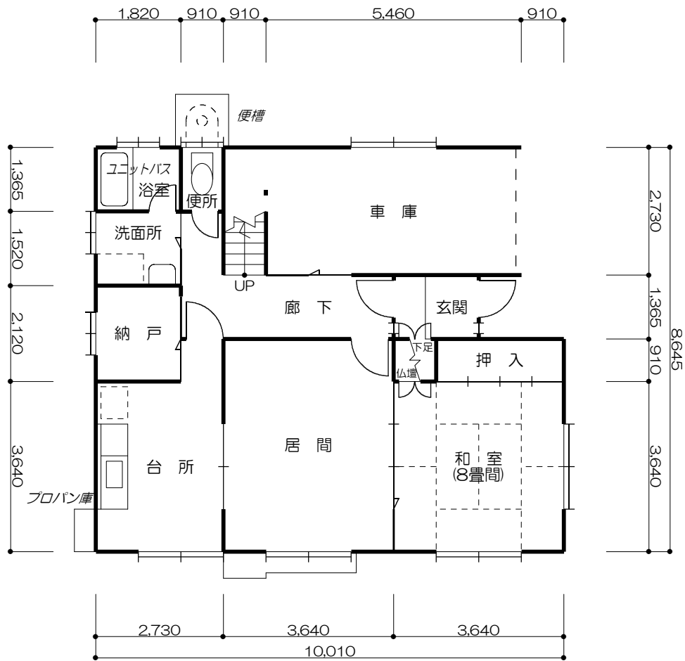
1 階 平 面 図
