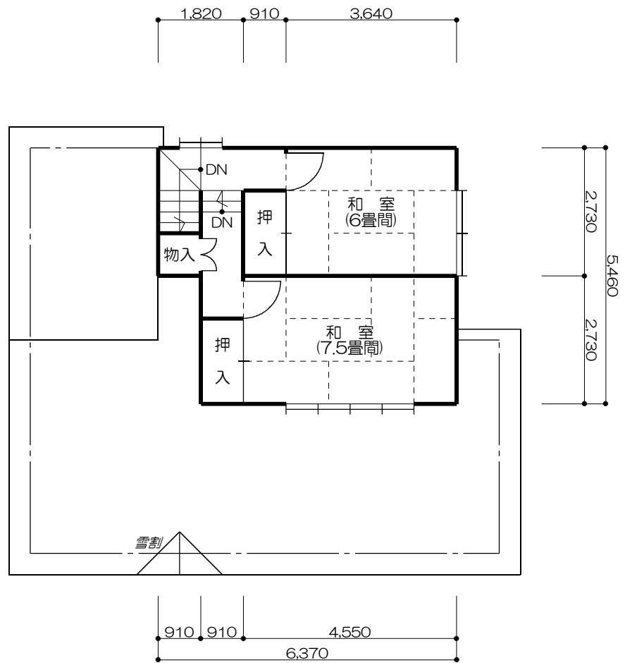
2 階 平 面 図
