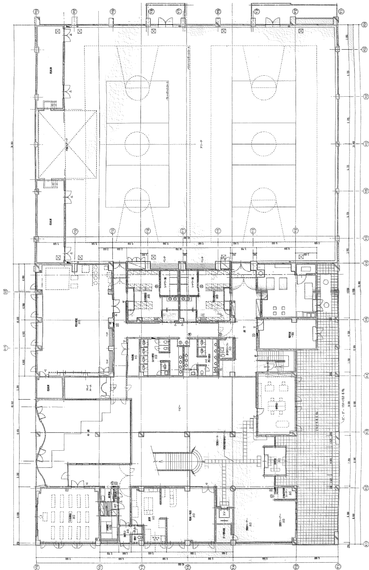
1階平面図
