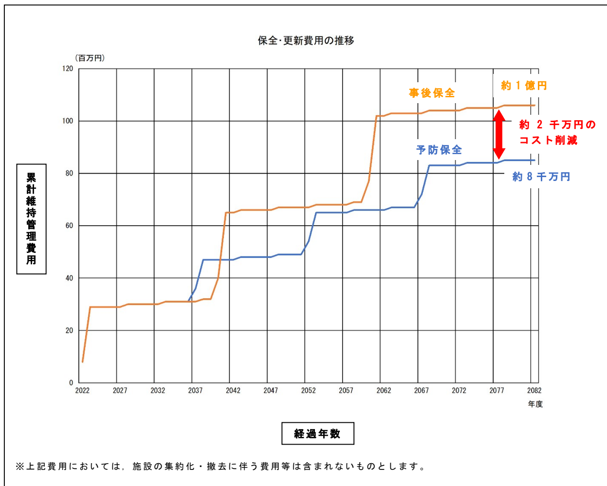
図6 保全・更新費用のシミュレーション
