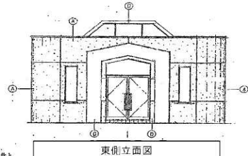
東側立面図
