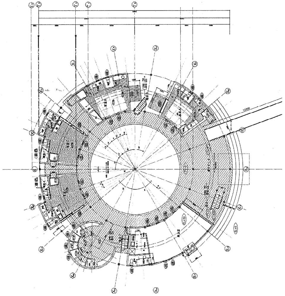
1 階平面図
