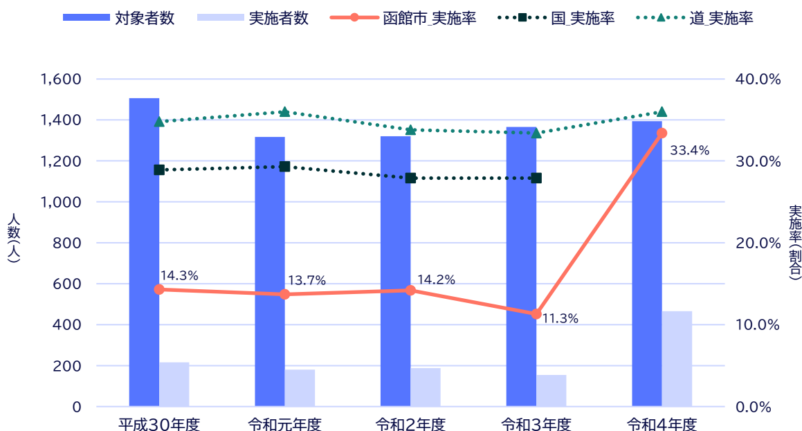
図表3-5-5-1：特定保健指導実施率（法定報告値）
