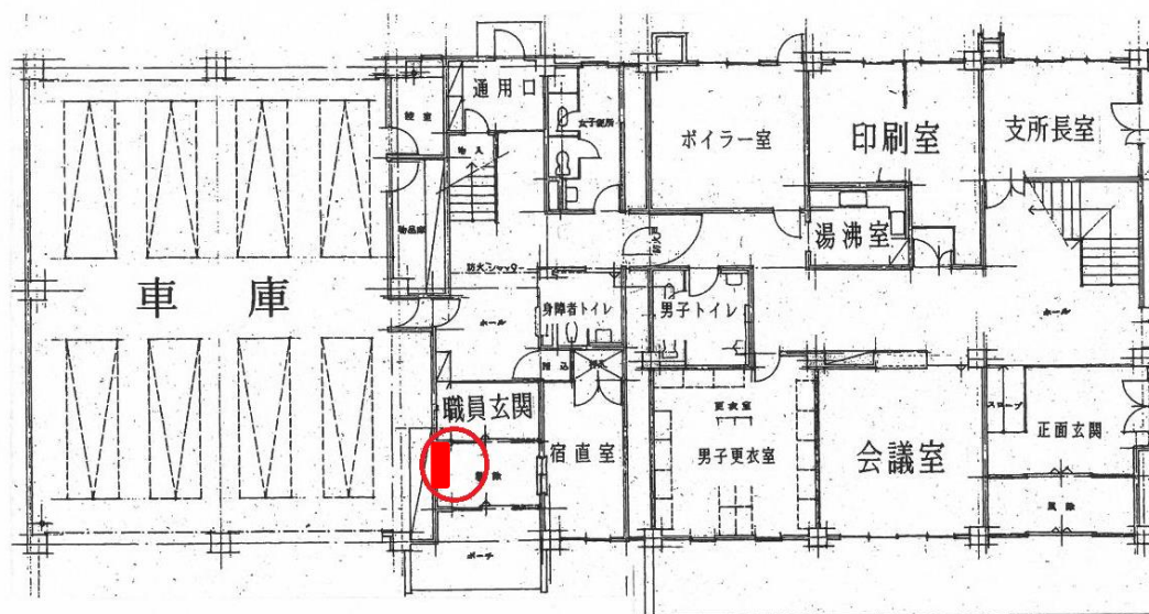
施設 1 階平面図
