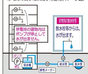
停電時の受水槽式給水の建物(イメージ図)
