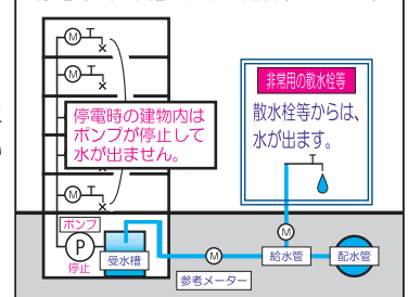
停電時の受水槽式給水の建物(イメージ図)
