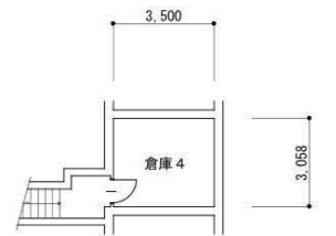
地階平面図 S=1:100
