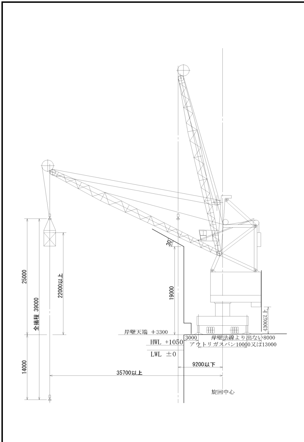
大型クレーン全体図
