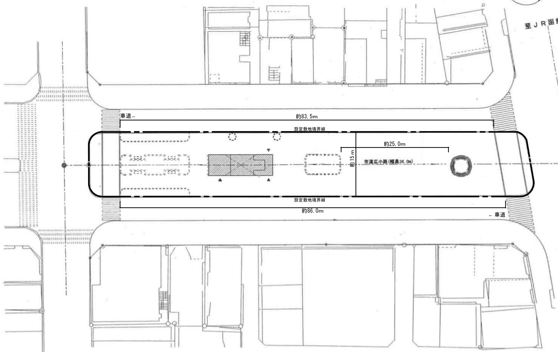
配置図 1 : 5 0 0
