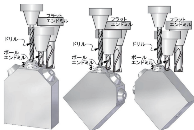
図2 3軸制御加工例
