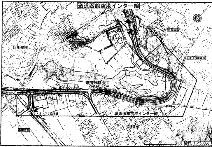
道道函館空港インター線（空港通）工事図
