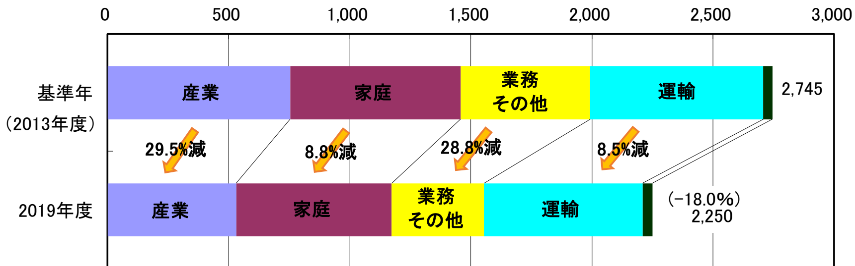
函館市の部門別CO 2 排出量(千t-CO 2 /人・年)
