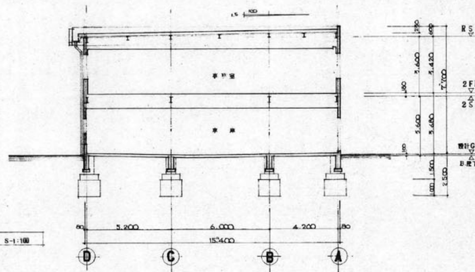
西立面図 S-1:100
