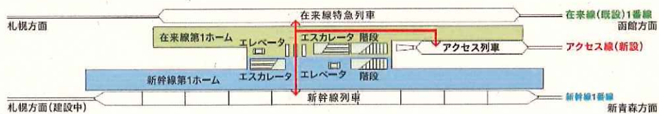
新函館北斗駅平面図
