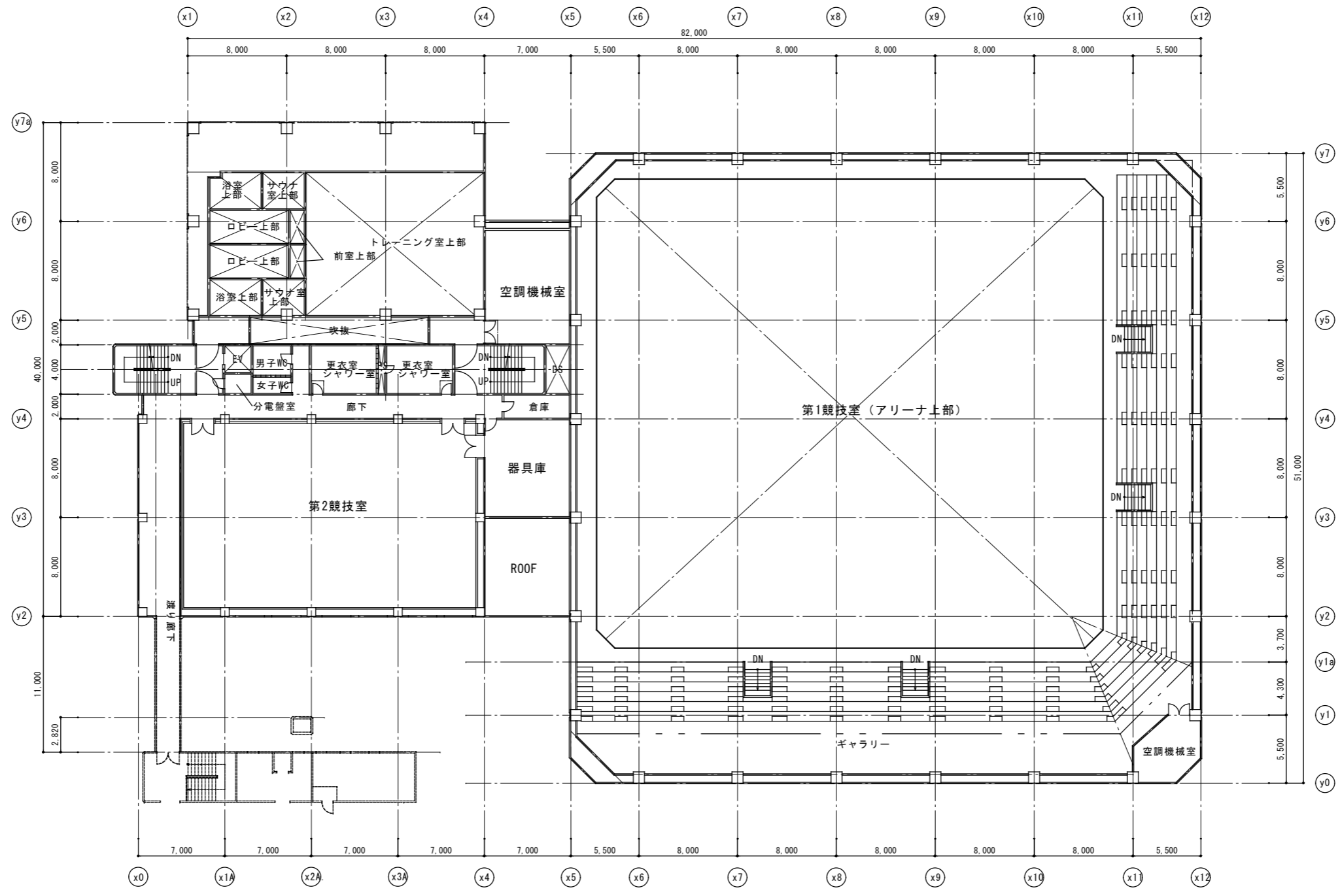
3階平面図 S=1:400
