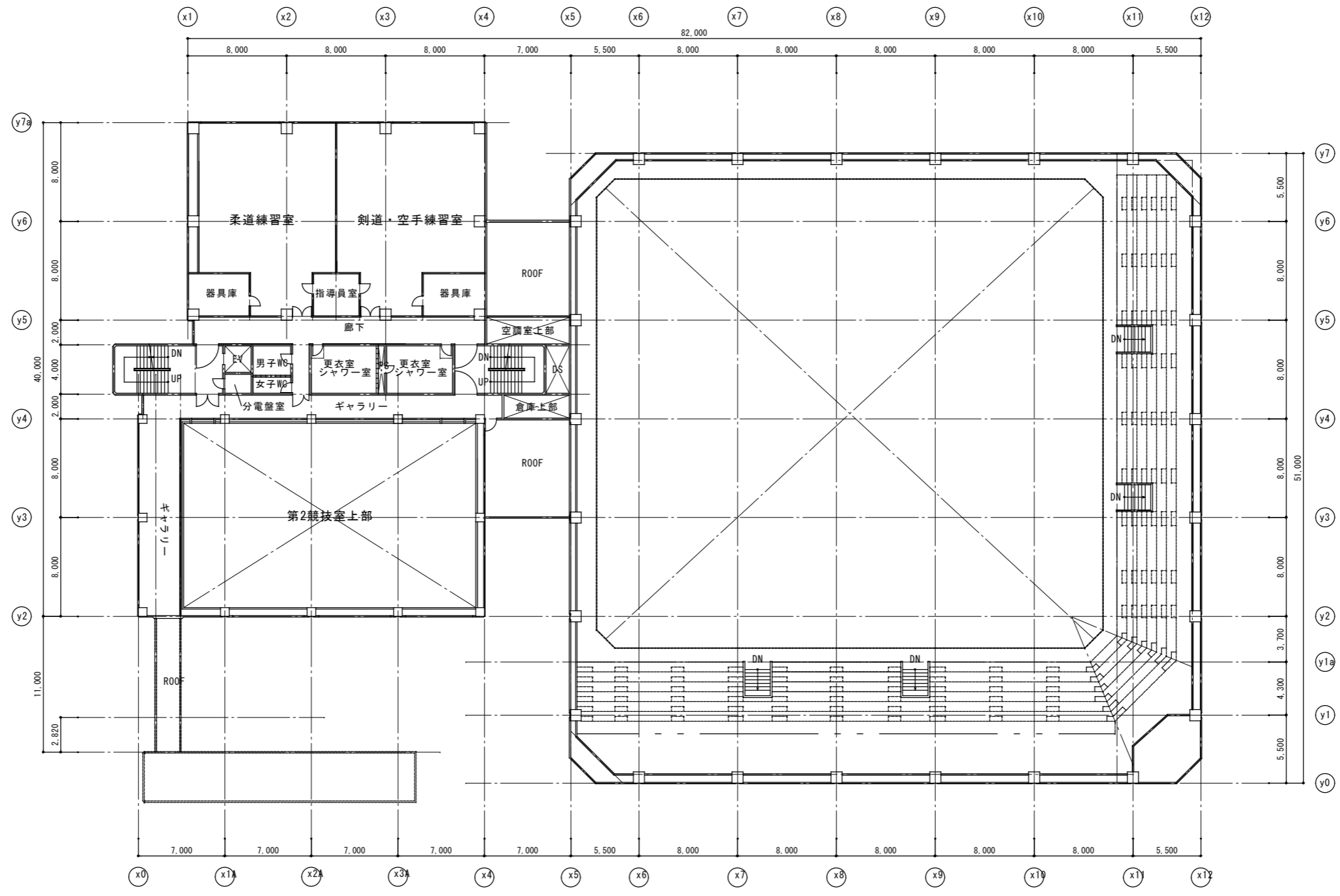
4階平面図 S=1:400
