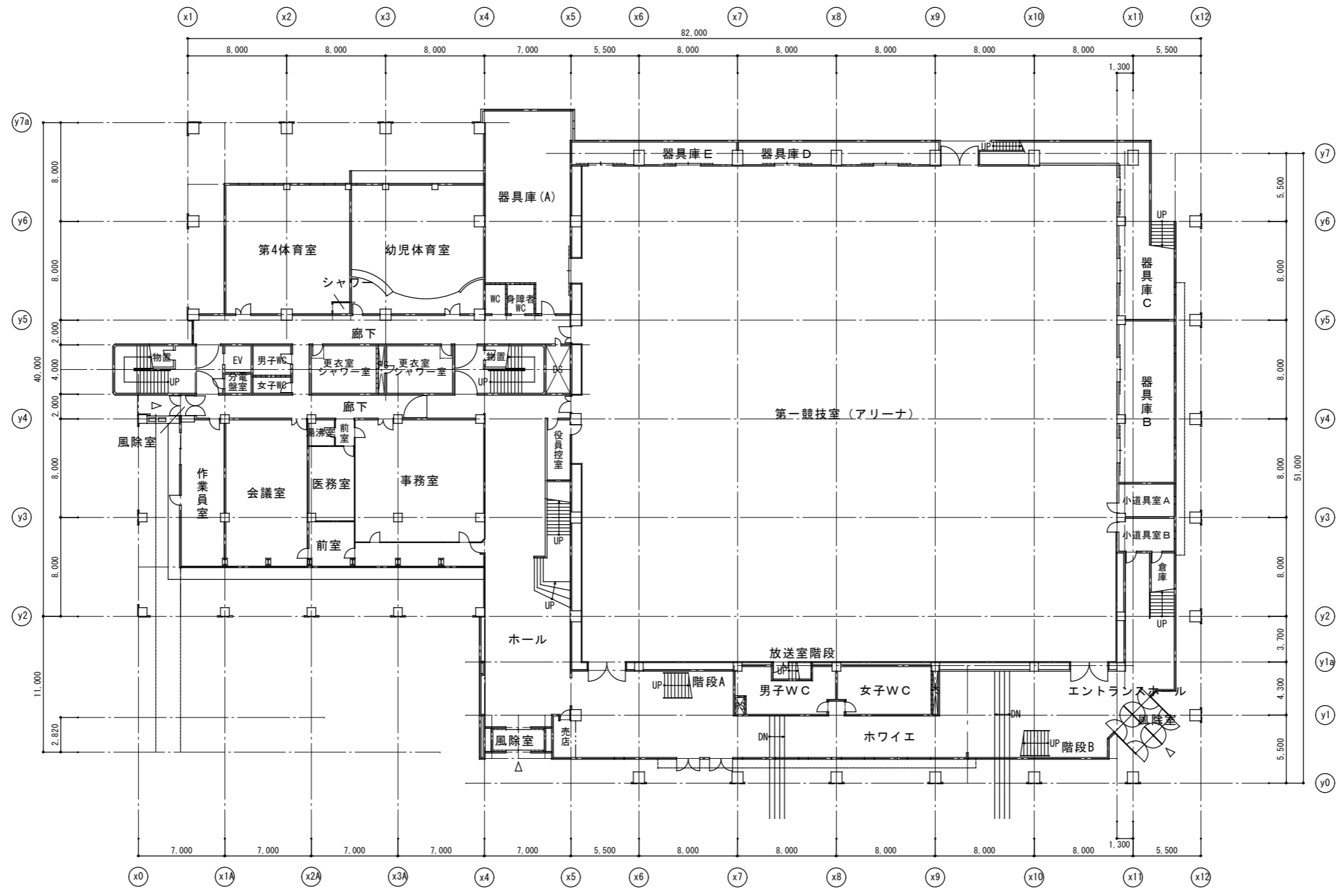
1階平面図 S=1:400
