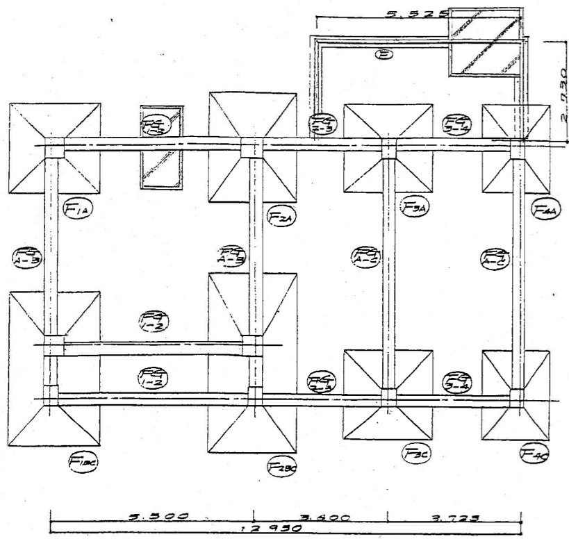
基础平面图 5:100
