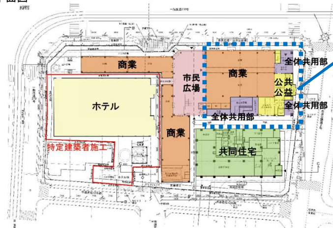
4.1階平面図
