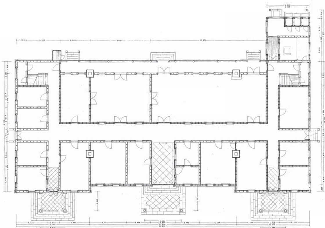
1 階平面図
