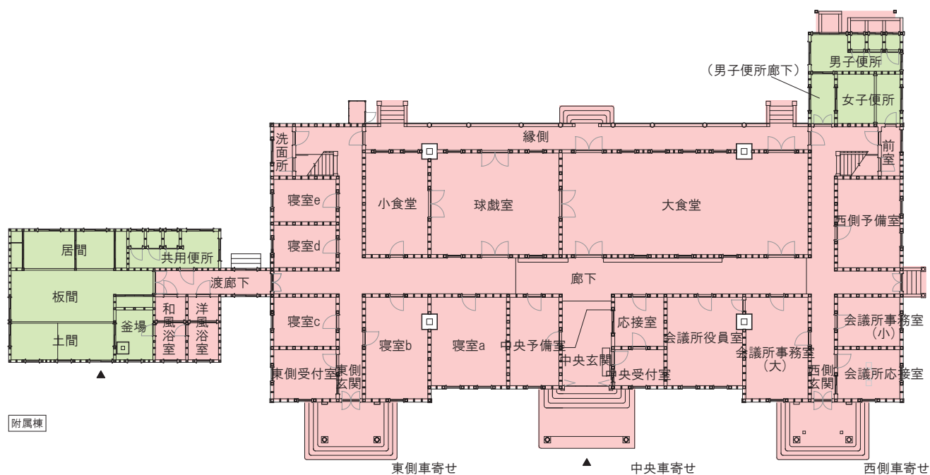
2階平面図
