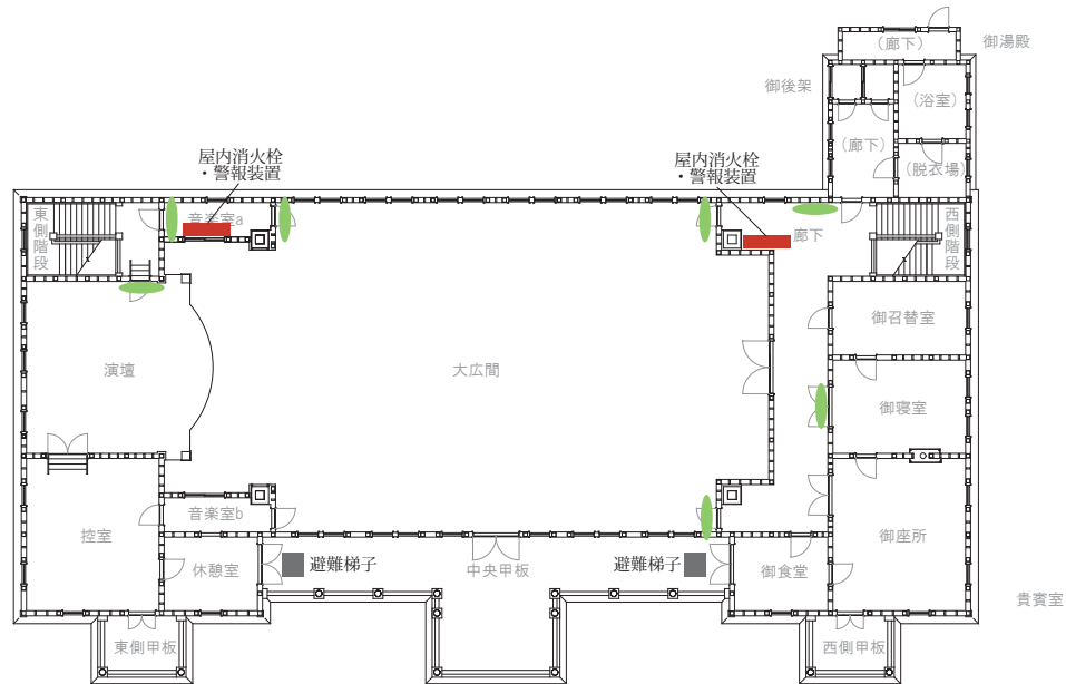
2階平面図
