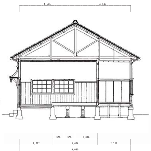
梁間断面図
