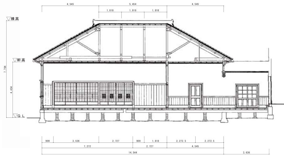
桁行断面図
