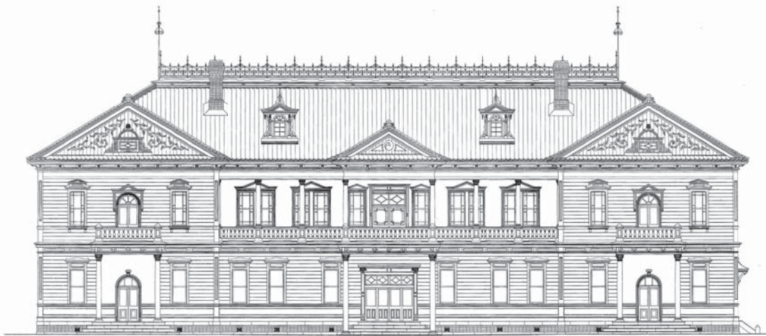
正面図（北）
