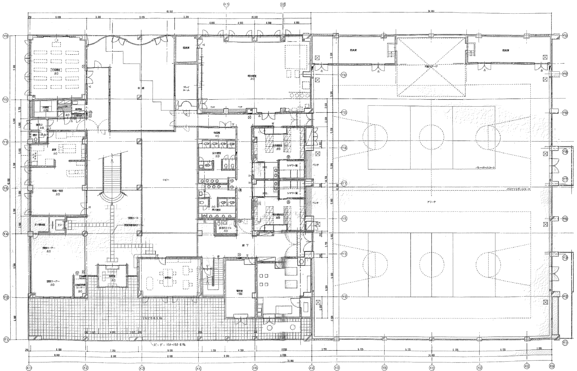
1階平面図
