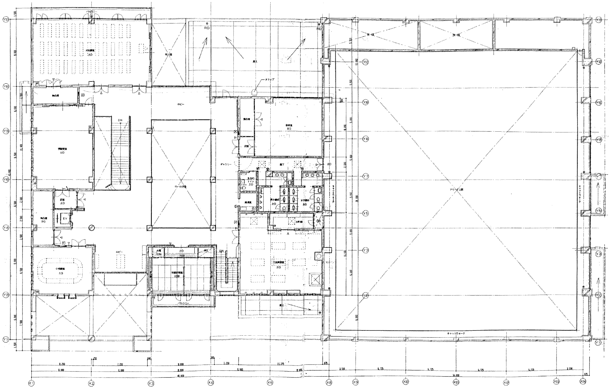
2階平面図
